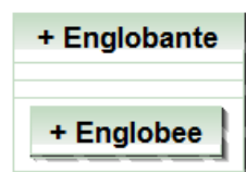
Figure 1.8. Classes imbriquées
