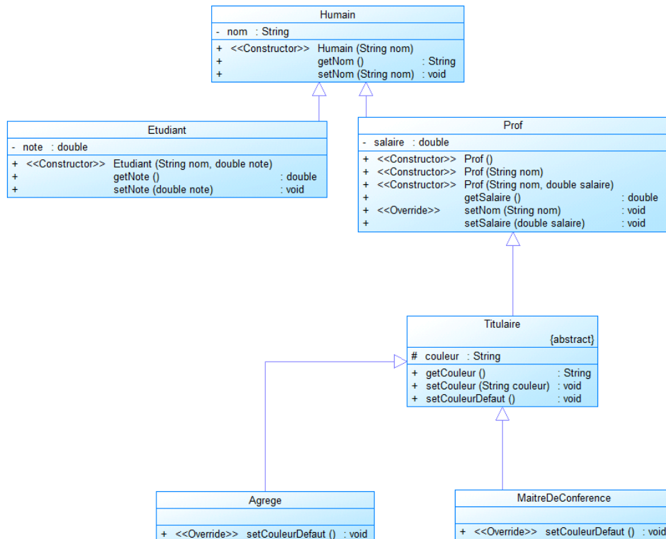
Figure 2.6. Arbre d'héritage
