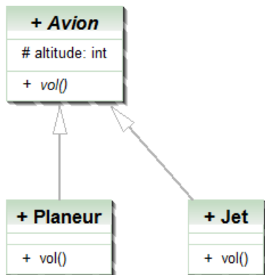
Figure 1.11. Classe Abstraite
