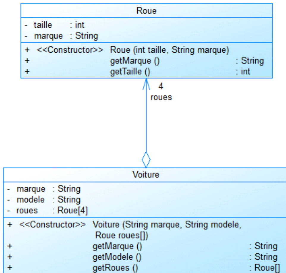
Figure 2.3. Agrégation partagée
